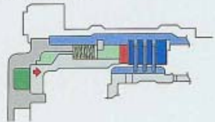
Lamellenbremse B1
